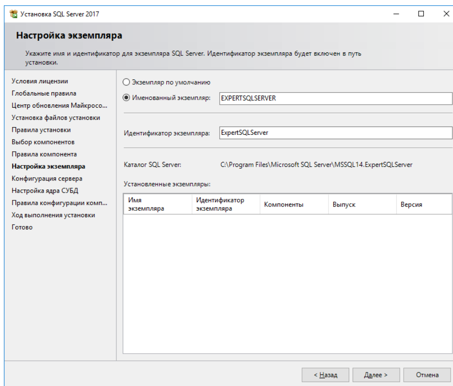
Рисунок 5.19 – Настройка экземпляра SQL Server
